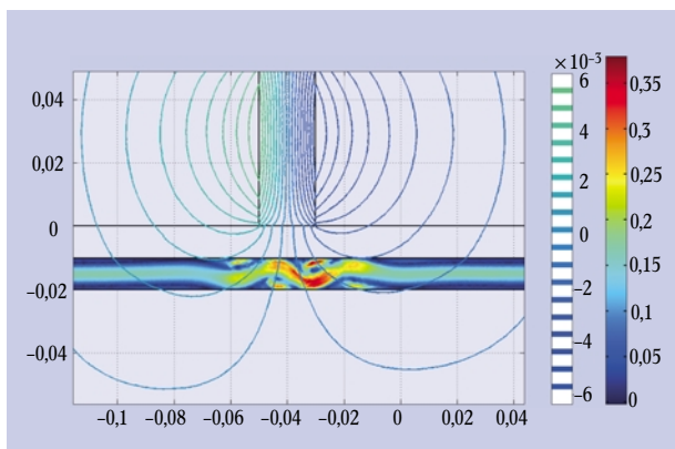
Abb. 2: Die Lösung des Problems zur Zeit t = 0,45 s. Der Surface-Plot zeigt das Geschwindigkeitsfeld (rechte Skala), der Contour-Plot das Vektorpotential (linke Skala).
