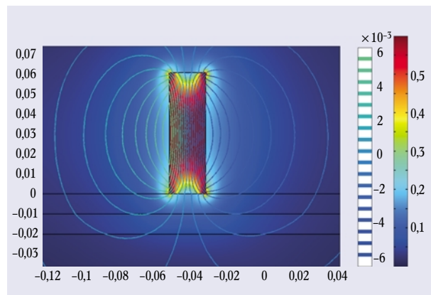
Abb. 1: Die mag. Flussdichte (Surface-Plot, rechte Skala) und das Vektorpotential (Contour-Plot, linke Skala).
